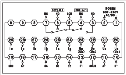
接线图请以实物机壳为主 注:电压输入接线端子,括号内标号表示三相三线接法;接线如有变动,请以出厂仪表接线为准。
